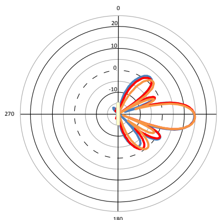
V-pol Elevation
